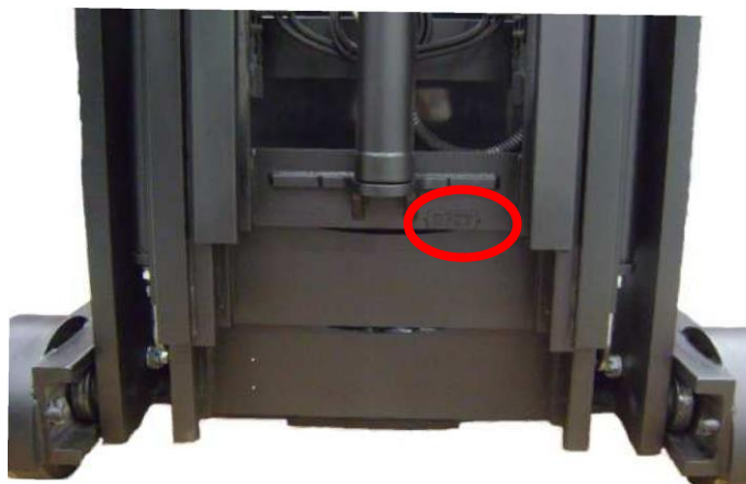
PLAQUETA DE Nº DE SÉRIE DA TORRE Eleva os garfos e verificar a plaqueta na travessa inferior.
